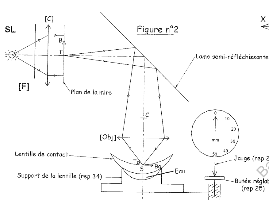
Figures n°2 et n°3 : Schémas des voies d'éclairage et de projection
